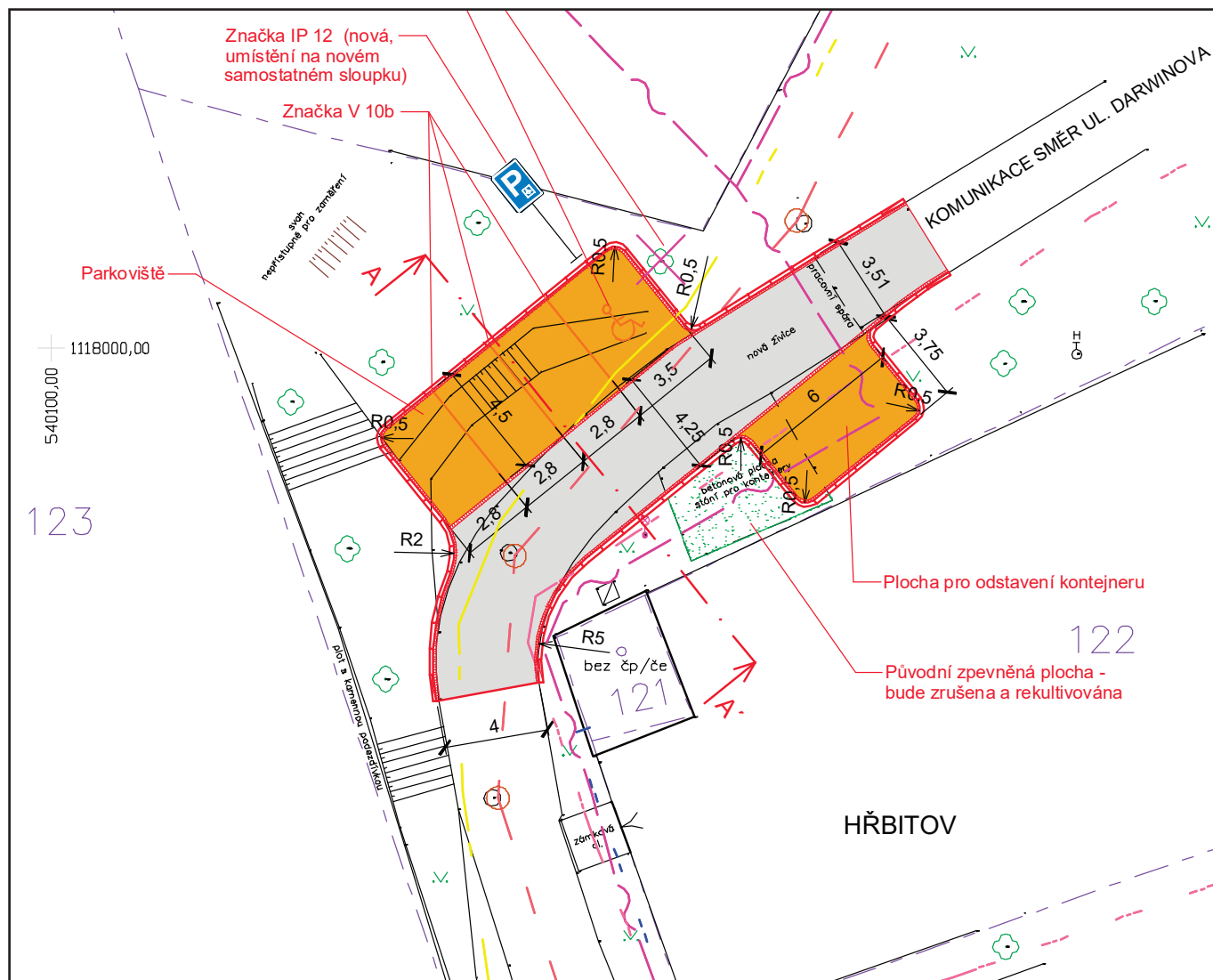
Sv. Kopeček, parkoviště u hřbitova: situace pozemní komunikace.
