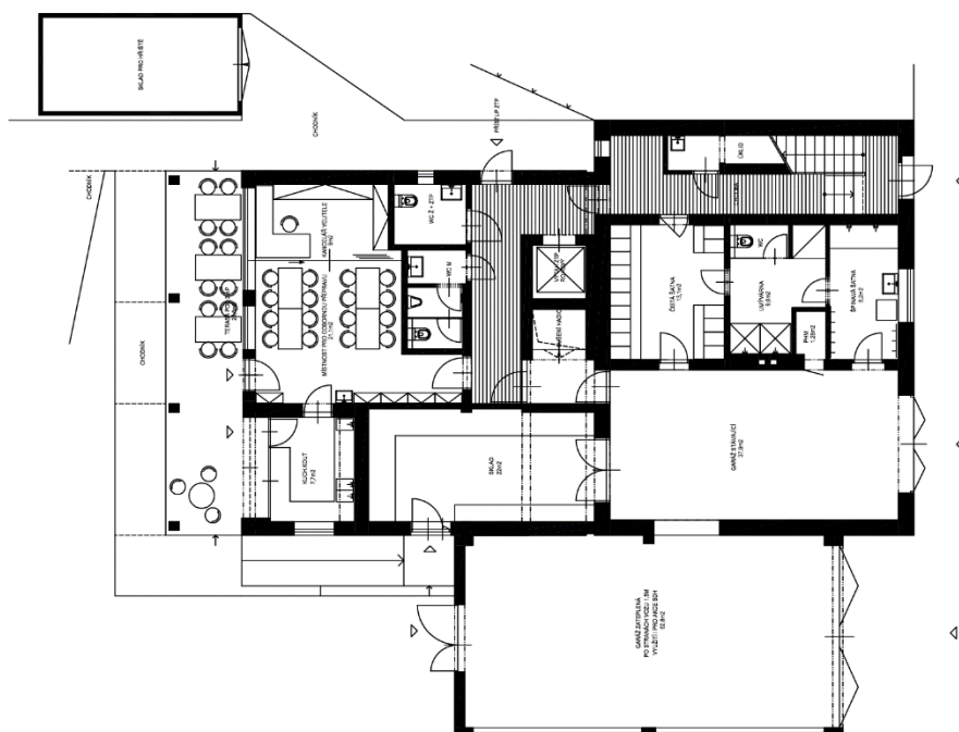
Půdorys přízemí (1.NP)
