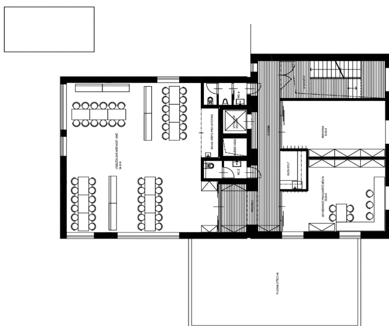
Půdorys 1. patra (2.NP)
