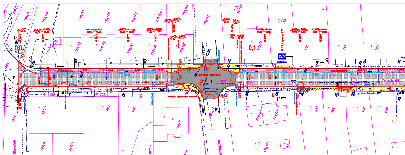
PARTYZÁNSKÁ – KOMUNIKACE (VÝŘEZ)
