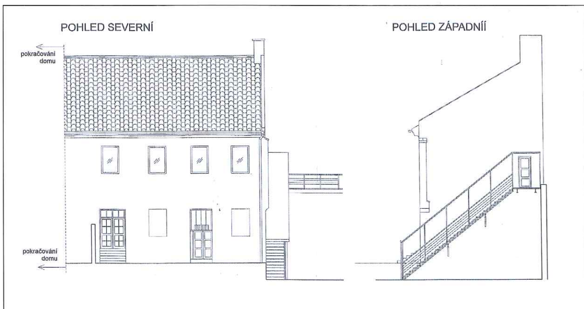
Výkres zaměření objektu na parcele 383/4 (Ing. Petr Štěpánek, 2011)
